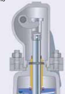
Кольцевой гаситель вибраций H4
