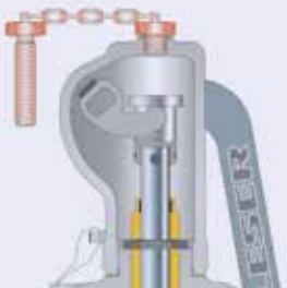
Блокировочный винт
