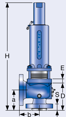
Конструкция с уравновешивающим сиффоном из нержавеющей стали
