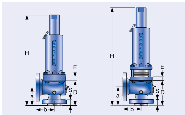
Стандартная конструкция
