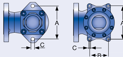
Opорные кронштейны
